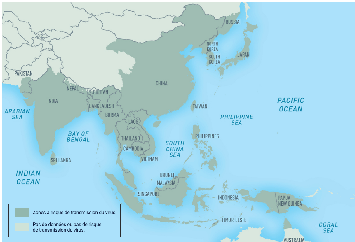
Figure. Zones de circulation du virus de l'encéphalite japonaise.
